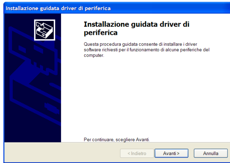
Abb. 6 – Treiberinstallation
