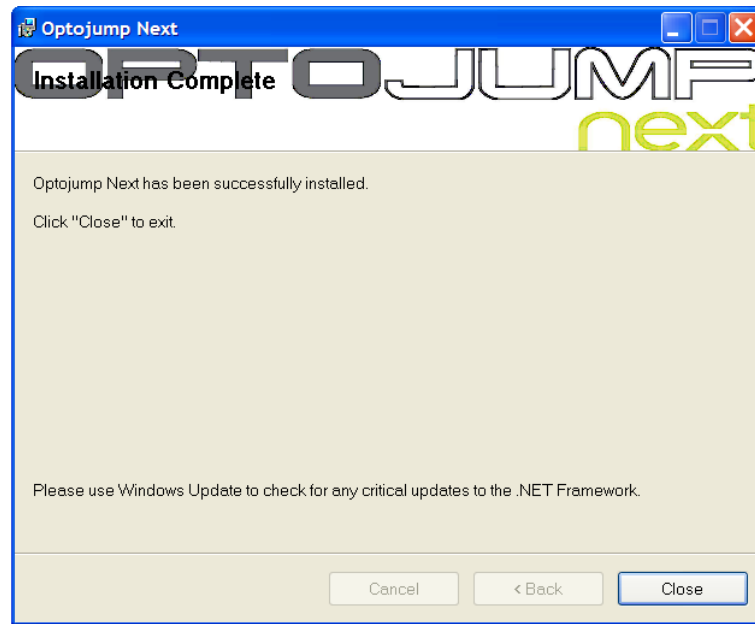
Abb. 8 – Installationsassistent - abgeschlossen
