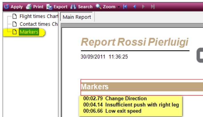
Abb. 77 - Druckbericht
