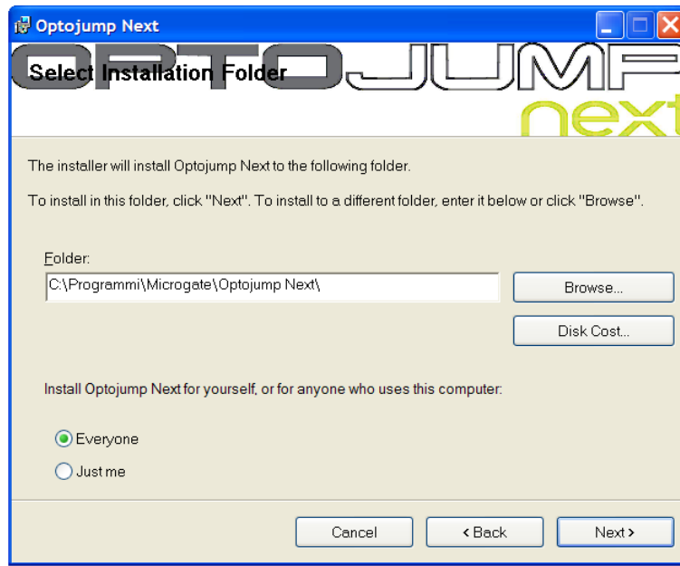
Abb.4 – Installationsassistent - Dateneingabe
