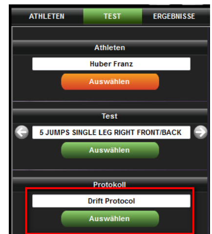
Abb. 110 - Protokollauswahl
