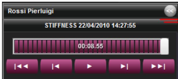
Abb. 57 – Geöffnetes Konfigurationsfeld
