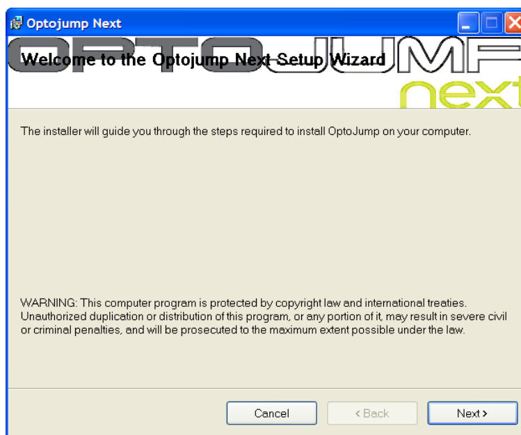
Abb. 3 – Installationsassistent - Willkommen
