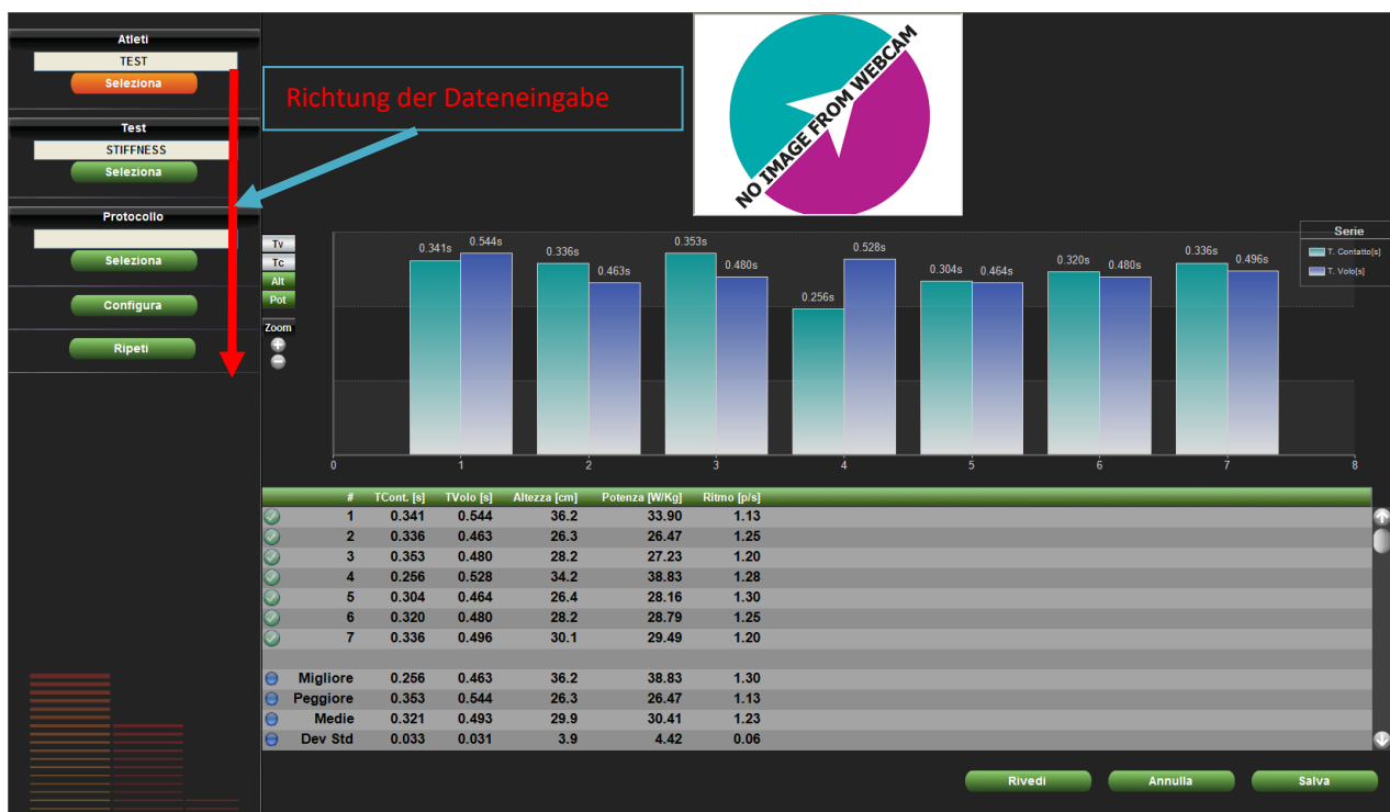
Abb. 30 - Ausführen
